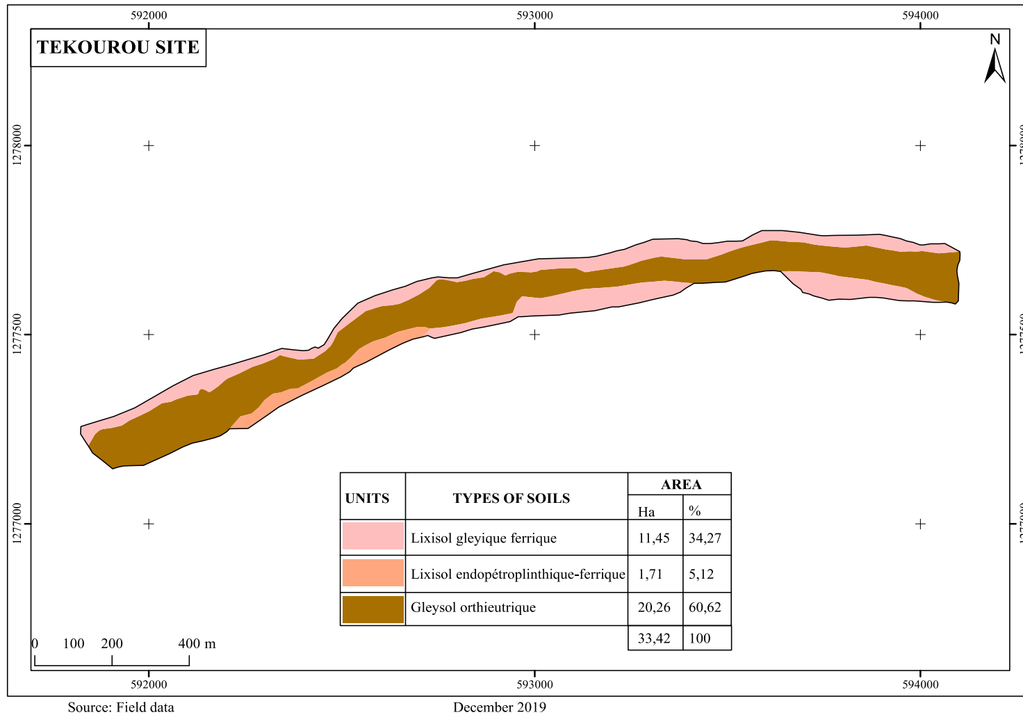
Fig. 3. Soils of Tékourou lowland
